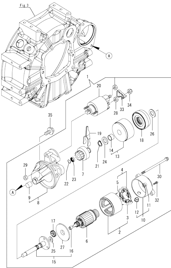
OCD50-M00540 3TNM74F-NHGE Fig.14. STARTER MOTOR
